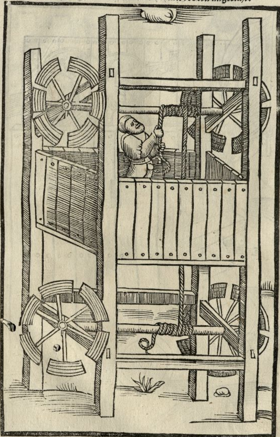
Ein Zuechthurn/vnden vnd oben mit redern angeeicht.
